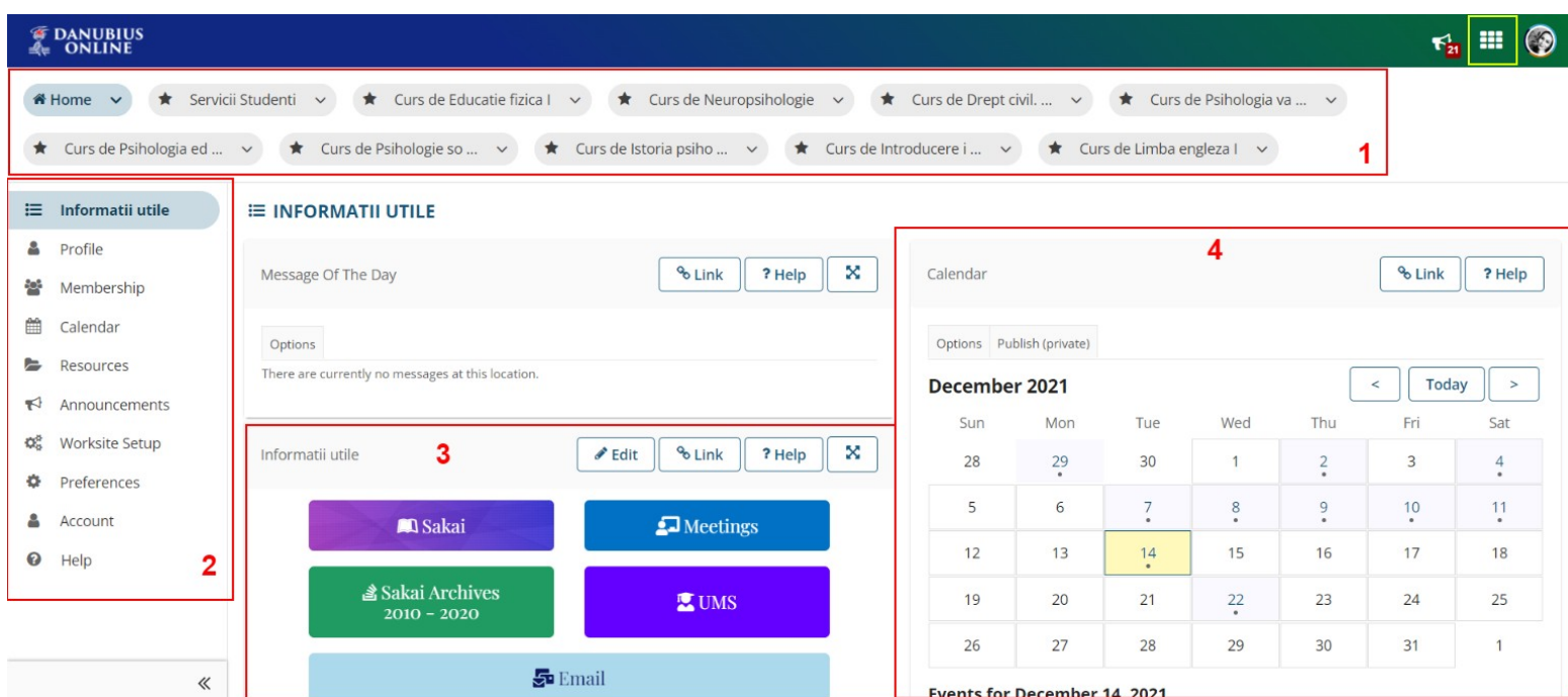
Figura 5. Fereastra utilizatorului
